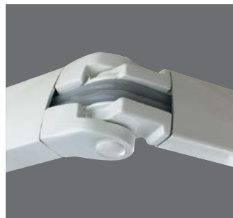
Modèle Grenat Jade Bras à double câbles gainés, testés à 20 000 cycles.
