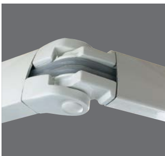
Bras testés à 20 000 cycles dotés d'une articulation à double câble gainé.
