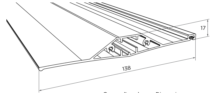
Coupe d'une lame - Dimensions en mm
