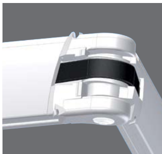
Modèle Grenat On'x. Bras Forty haute résistance, testés à 60 000 cycles.
